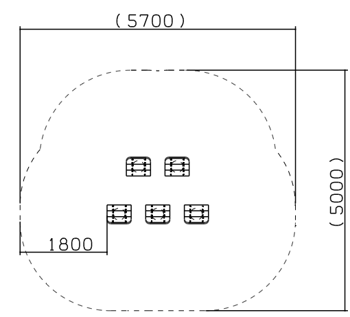
安全領域図 S=1/100 遊具の外形からあらゆる方向に 1800mmを安全領域とする。
