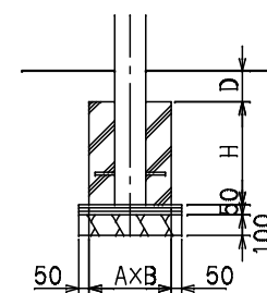
基礎詳細図
