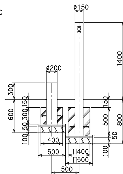
A-A矢視図
