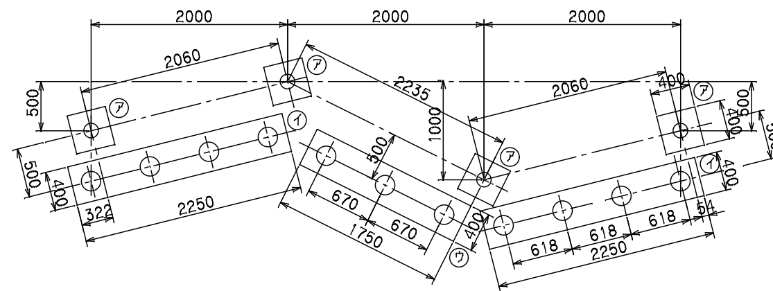
基礎伏図
