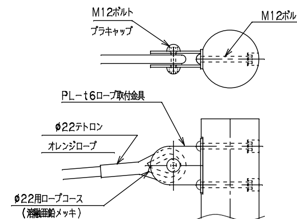
ロープ取付部詳細図 S=1/10
