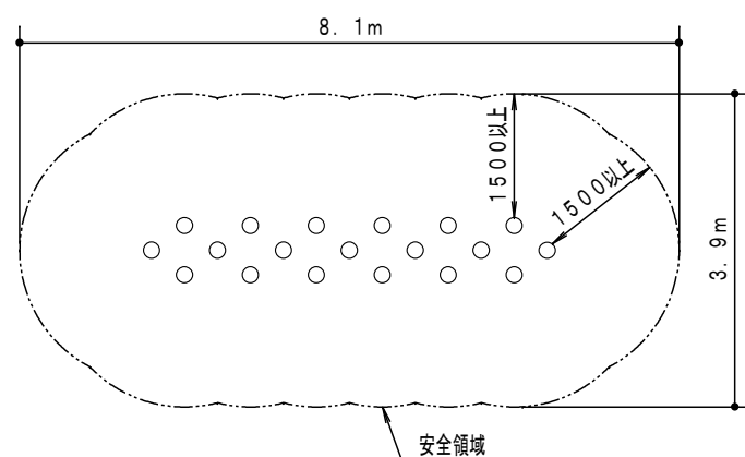
安全領域 平面図 1/100 (19本組設置例)
